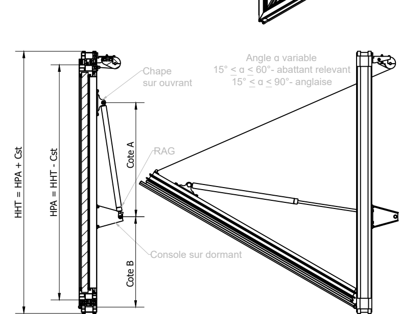
B-B ( 1:10 )
